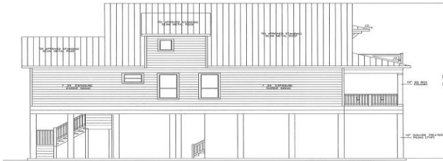
RIGHT ELEVATION SCALE: 1/8" = 1'-0"
